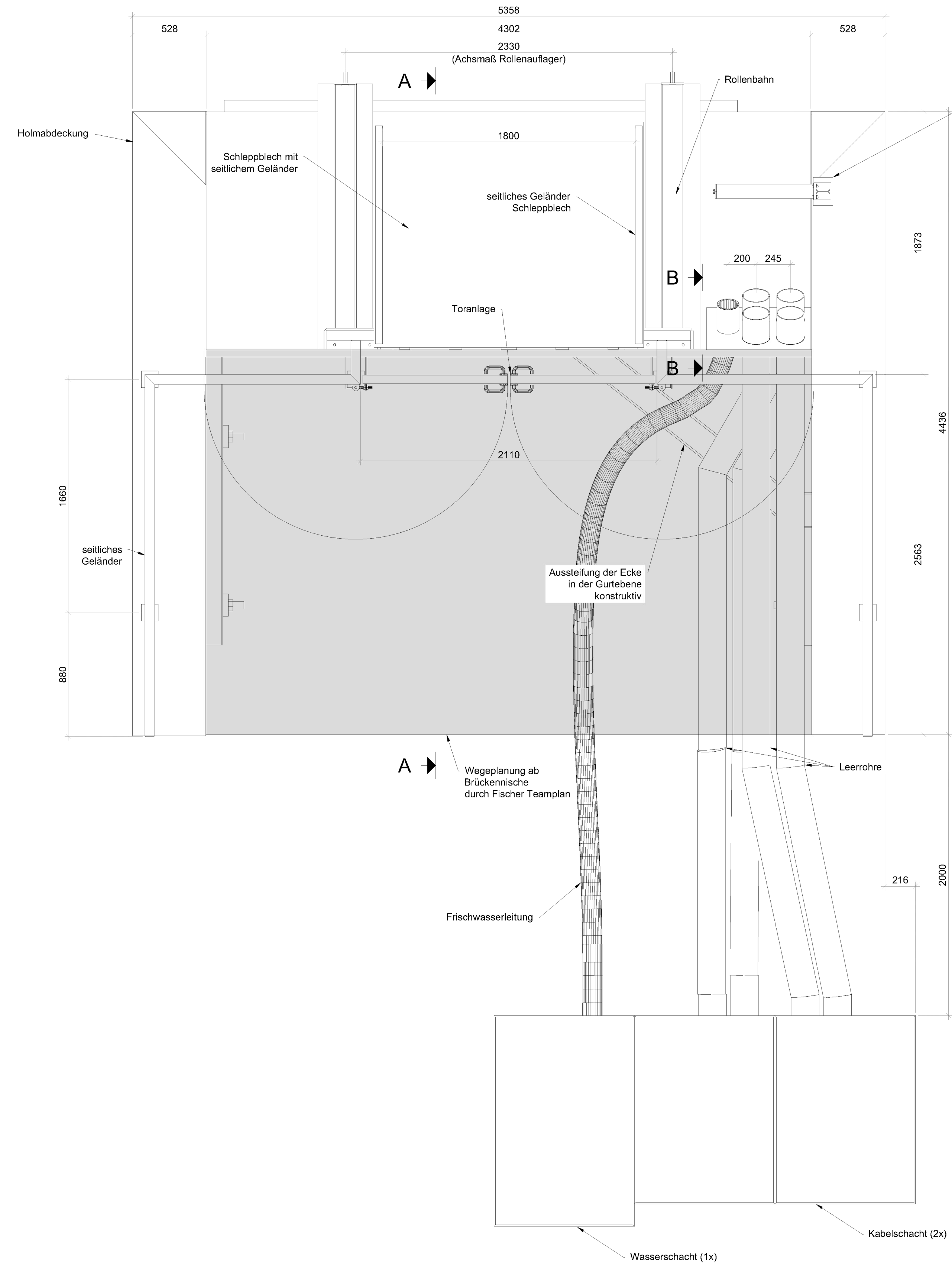
Draufsicht 1:20
