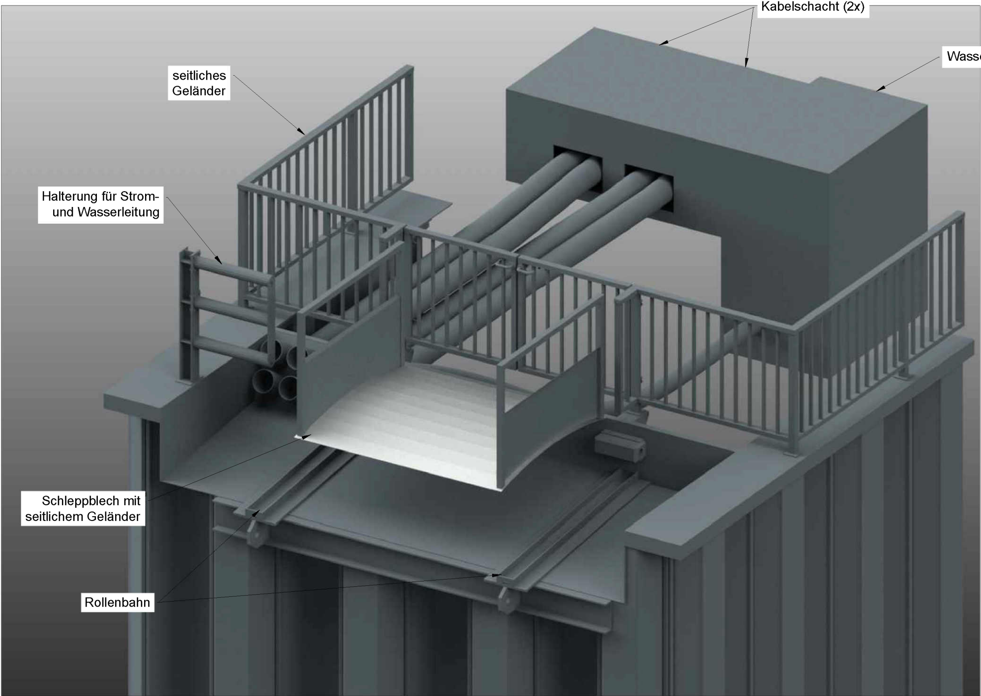
Isometrie Brückenaufleger
