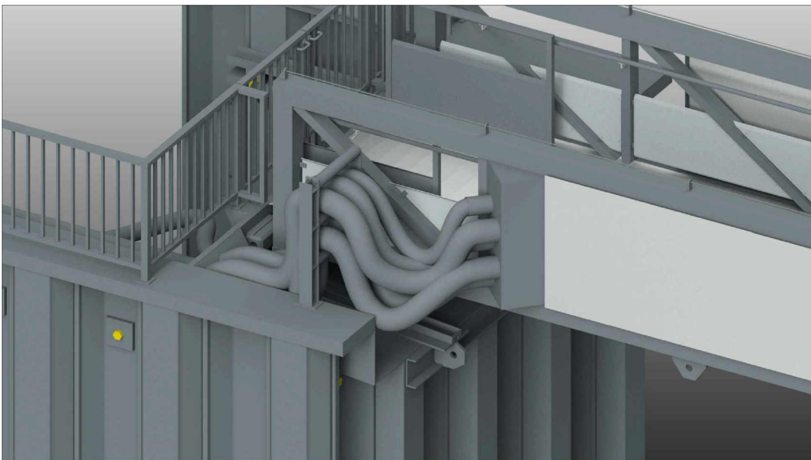
Kabellehrrohre zw. Brückenaufleger und Brücke
