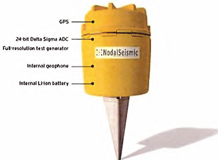
Abbildung 2: Kabelloses Geophon (Quelle: Bundesverband Geothermie).
