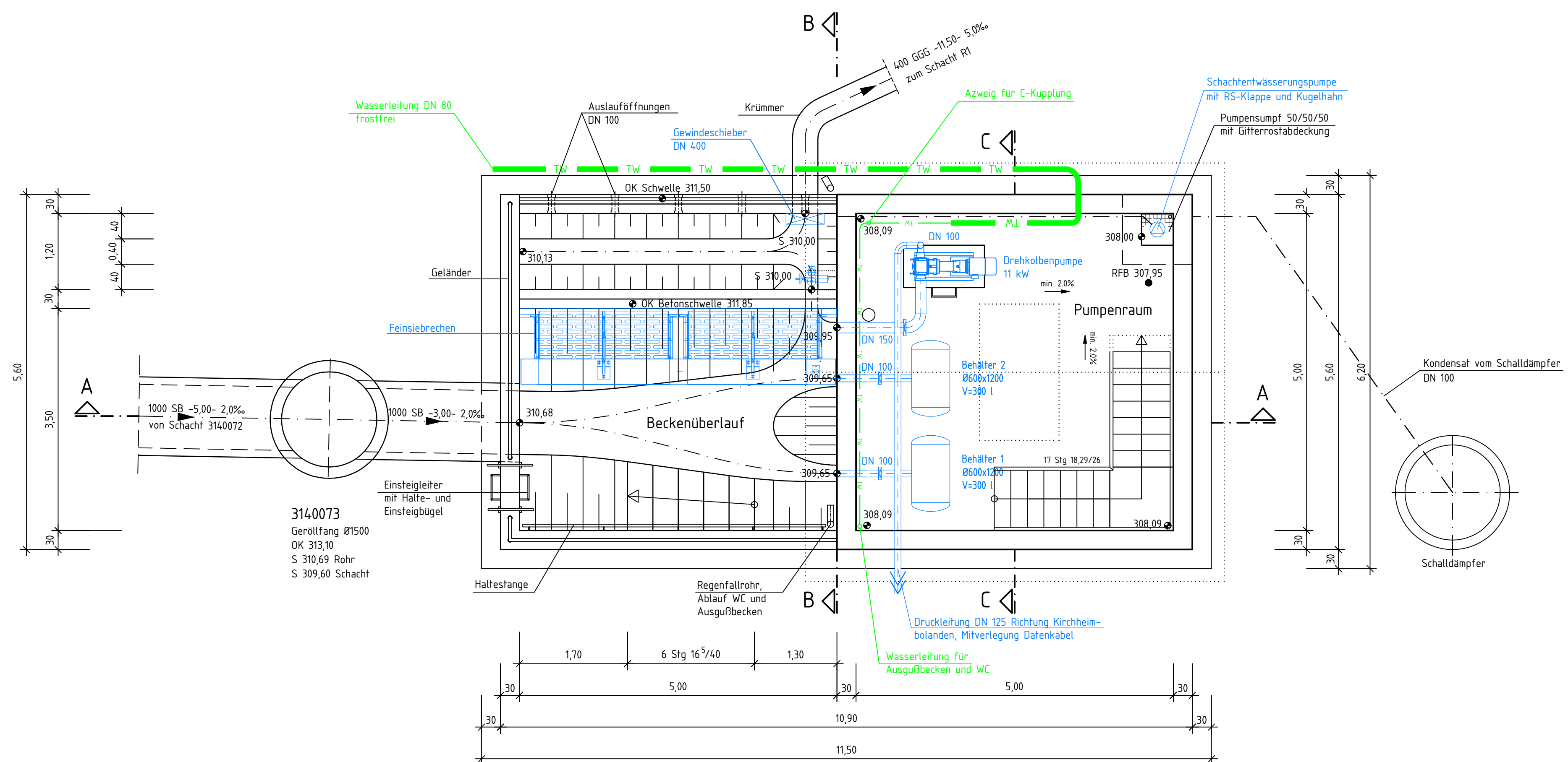
Grundriss 2 Beckenüberlauf und Pumpenraum
