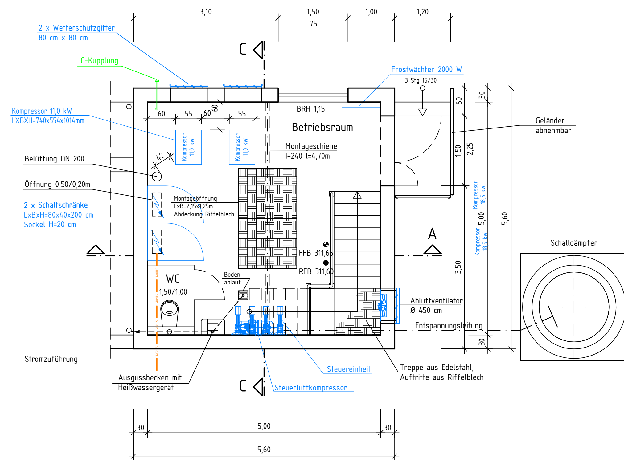
Grundriss 1 Betriebsraum
