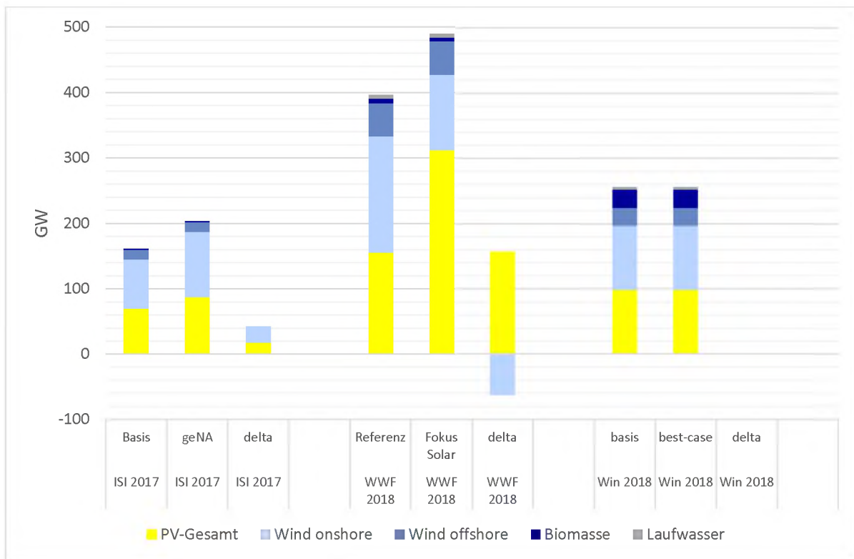
Abbildung 4-1: Installierte EE-Leistung im Jahr 2050 für drei ausgewählte Szenariopaare
