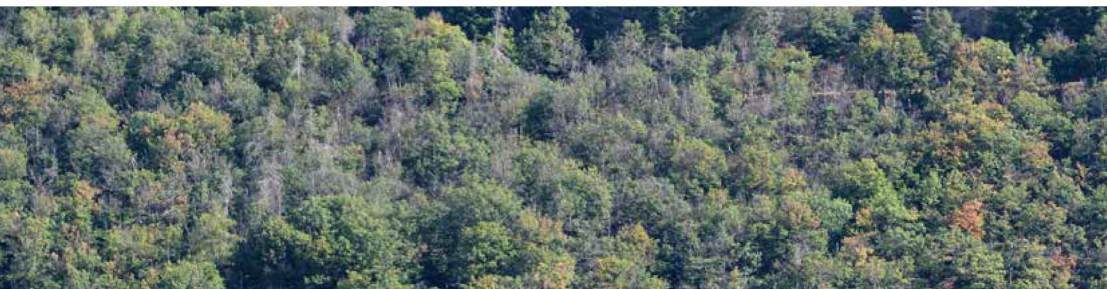
Geschädigter Trockeneichenwald im Forstamt Kirchheimbolanden Anfang September 2019 (oben) und zum gleichen Zeitpunkt 2020 (unten)
